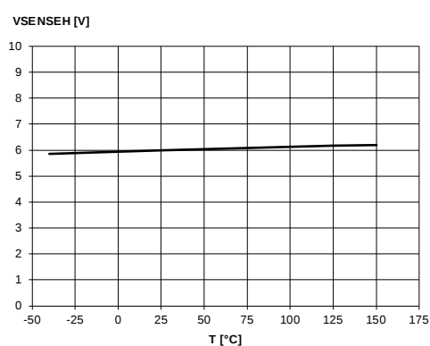
Figure 27: Vsenseh vs. Tcase
