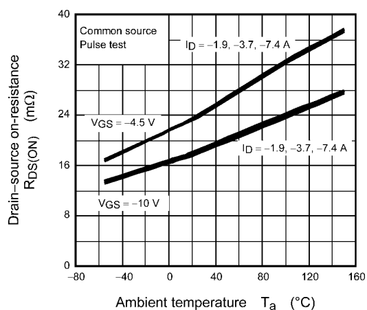
Fig. 8.1.6 R_{DS(ON)} - T_a
