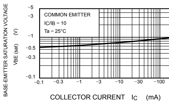
V_{BE(sat)} - I_C
