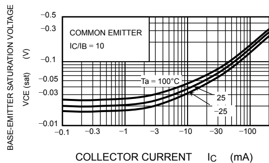
V_{CE(sat)} - I_C
