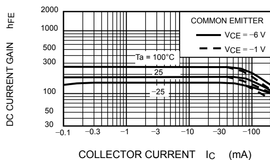
h_{FE} - I_C
