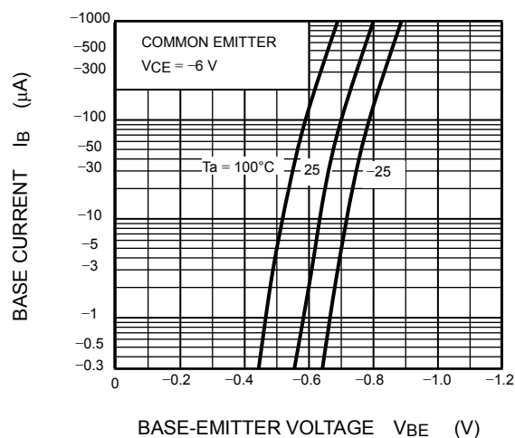
I_B - V_{BE}
