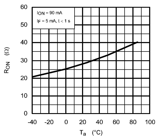
Fig. 14.5 R_{ON} - T_a
