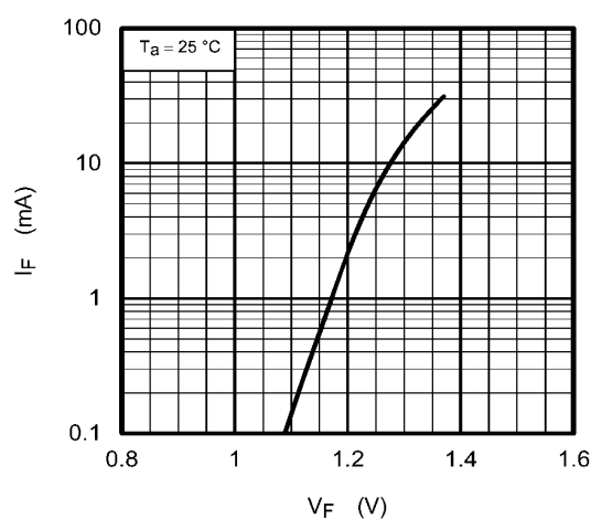
Fig. 14.3 I_F - V_F
