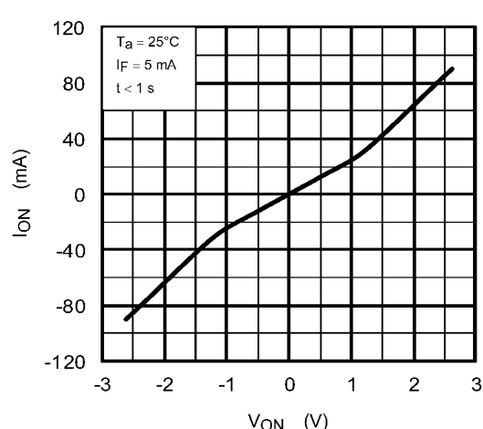
Fig. 14.4 I_{ON} - V_{ON}
