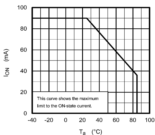
Fig. 14.2 I_{ON} - T_a
