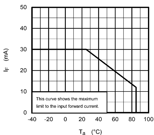
Fig. 14.1 I_F - T_a
