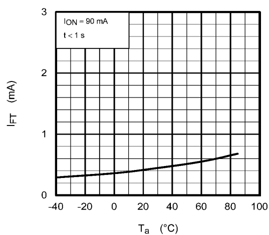
Fig. 14.6 I_{FT} - T_a
