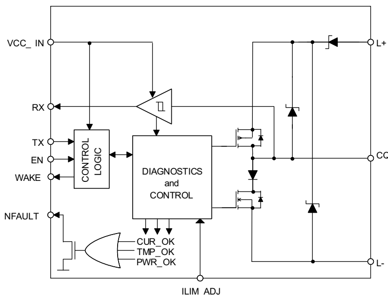
Figure 11. Block Diagram TIOL111
