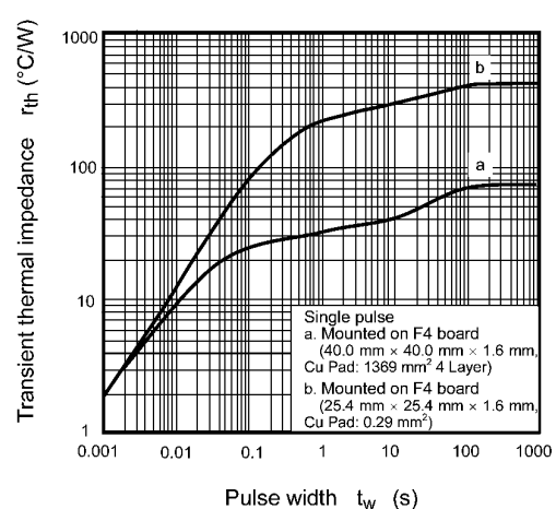
Fig. 7.12 r_{th} - t_w
