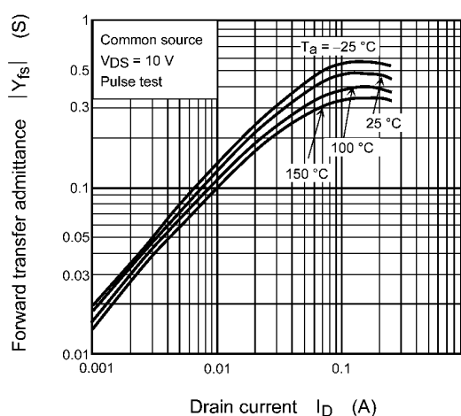
Fig. 7.8 |Y_{fs}| - I_D
