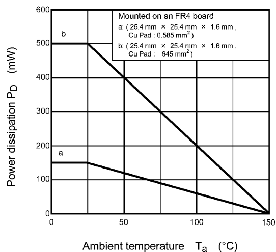
Fig. 7.11 P_D - T_a
