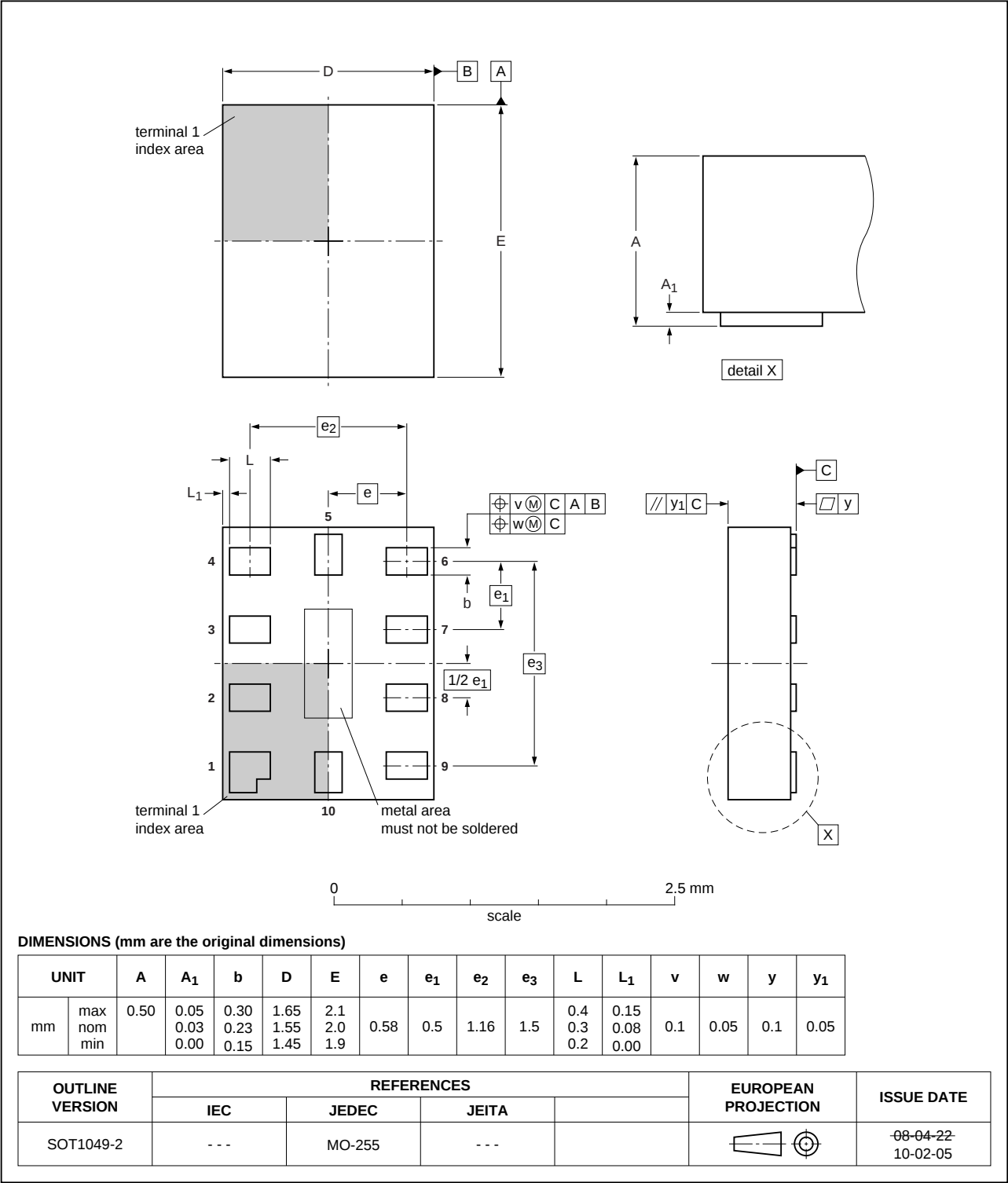
Fig 24. Package outline SOT1049-2 (XQFN10U)
