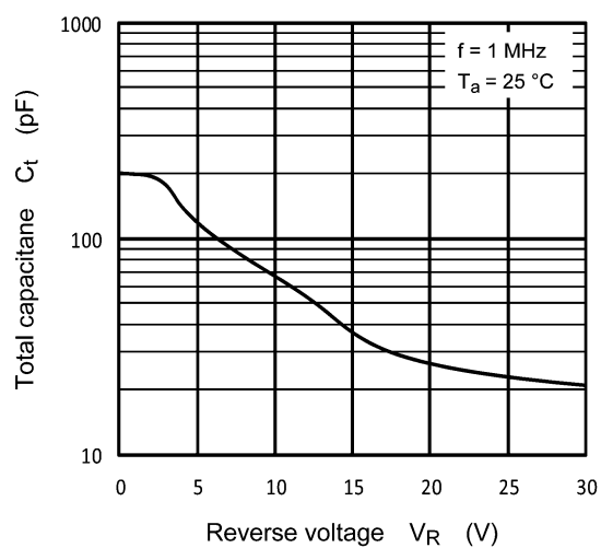
Fig. 9.3 C_t - V_R
