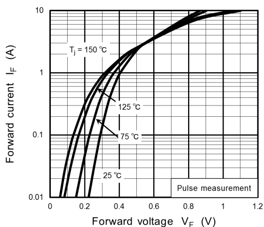
Fig. 10.1 I_F - V_F
