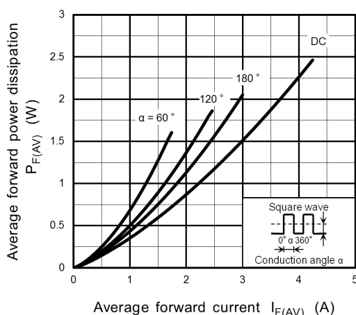
Fig. 10.2 P_{F(AV)} - I_{F(AV)}
