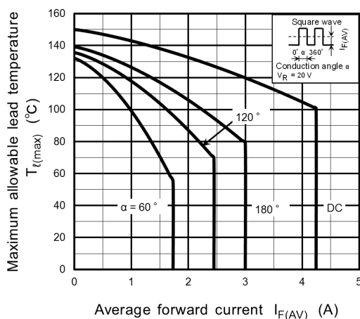
Fig. 10.4 T_{l(max)} - I_{F(AV)}
