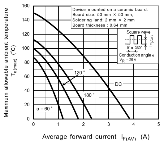
Fig. 10.3 T_{a(max)} - I_{F(AV)}
