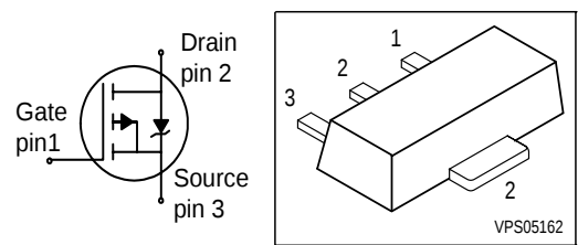
PG-SOT89
