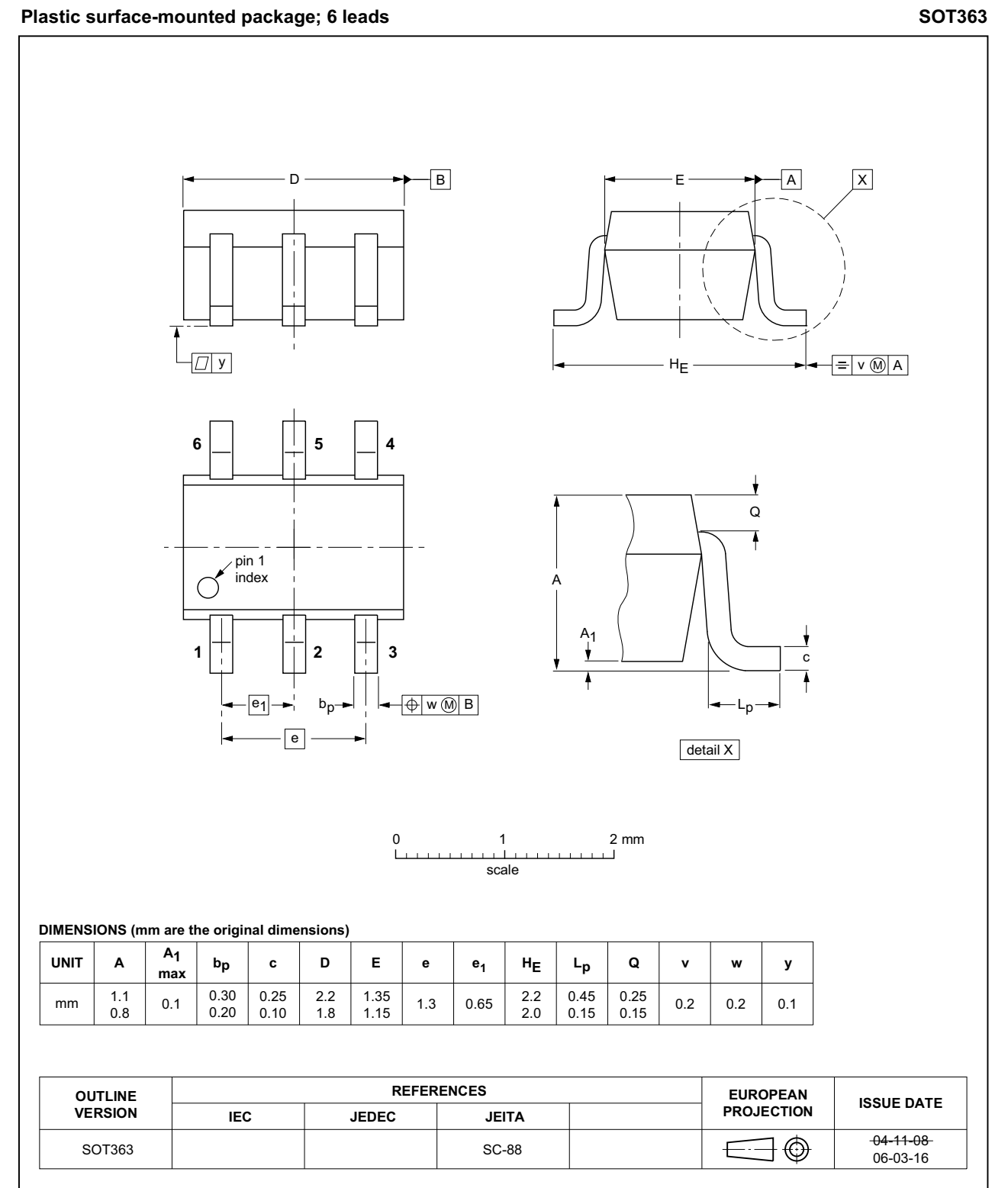
Fig 25. Package outline SOT363
